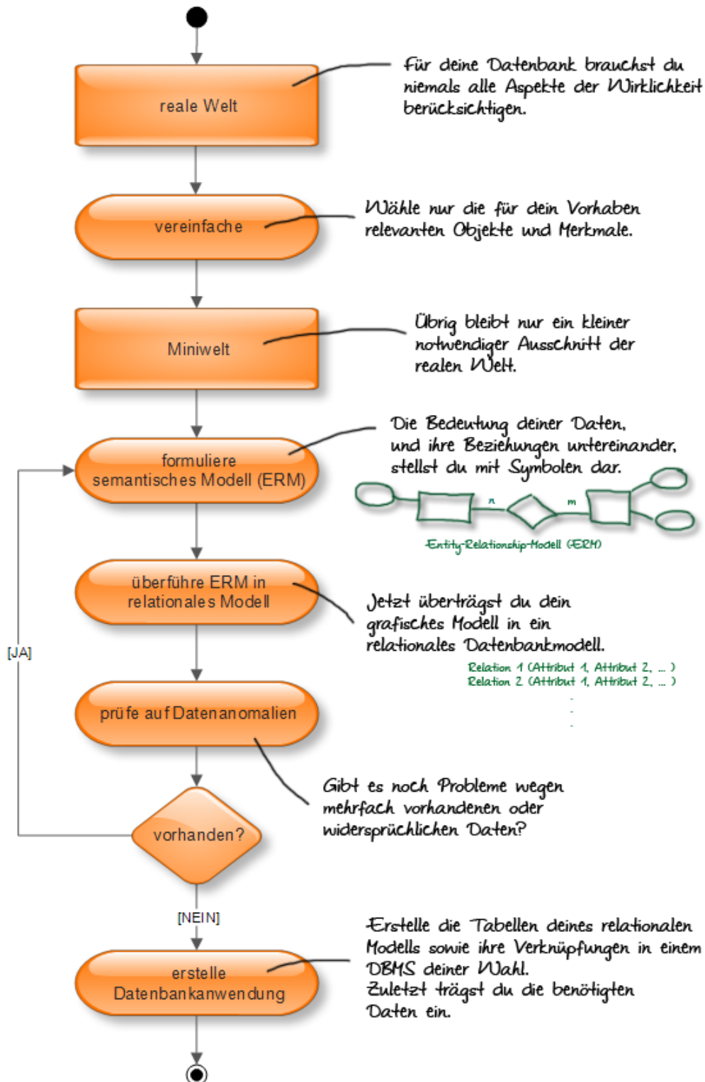
Abb. 01: Aktivitätsdiagramm zur Datenmodellierung
